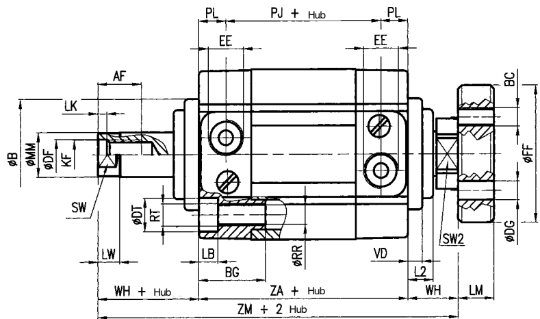
Masse
