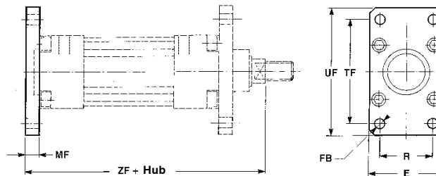
Hintere Montage
