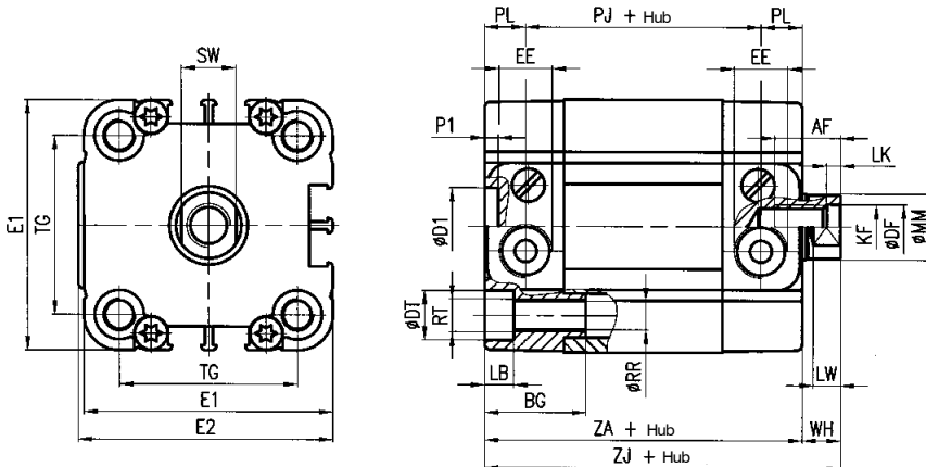
Masse RP 200...
