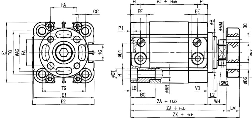
Masse RQ 200...
