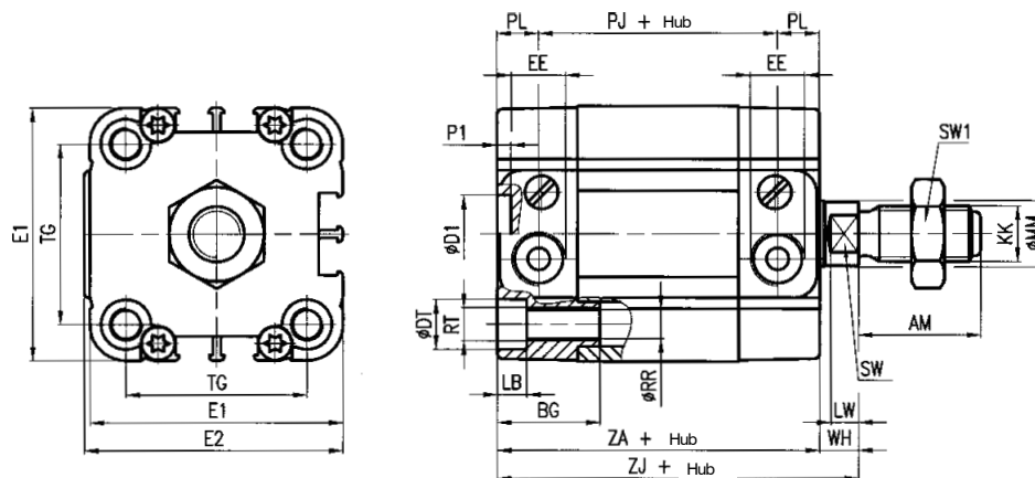
Masse RP 400...
