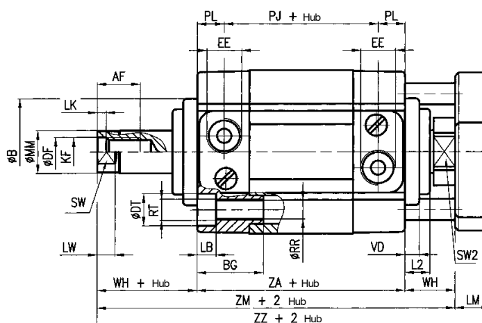
Masse
