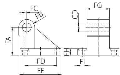
Schwenkbefestigung KF 19040-80
